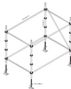
Tres elementos Básicos: Verticales TV, Horizontales TH y Base Regulable. Estructuración Modular
