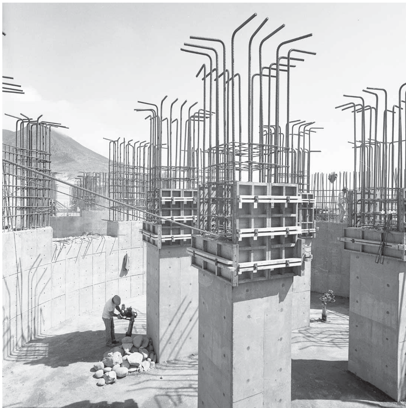
Pilares de hormigón armado en la planta de pellets de Huasco, 1978.
