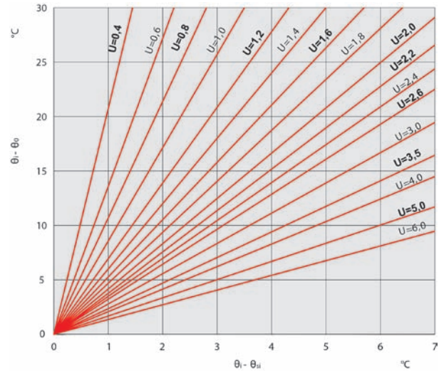
Figura 3.4. Ábaco utilizado para determinar la temperatura superficial interior de elementos verticales con flujo horizontal. (Fuente: CDT, 2012).
