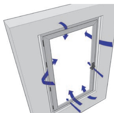
Figura 8.12: Principales puntos de infiltración de aire en ventanas abatibles.
