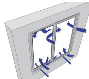
Figura 8.14: Principales puntos de infiltración de aire en ventanas correderas.
