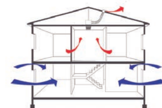
Figura 1.7: Esquema de infiltración por sistemas mecánicos de ventilación.
