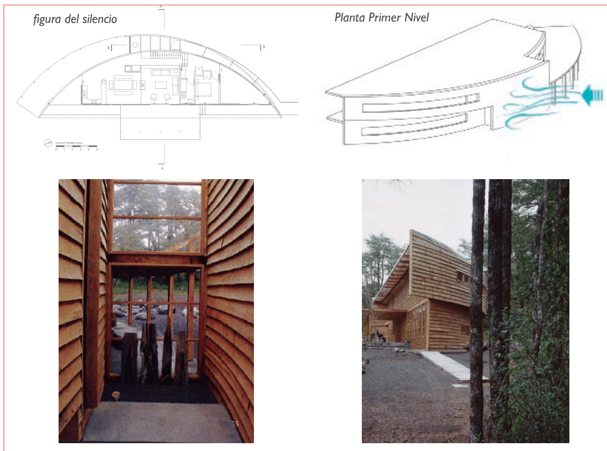
Figura 8.5: Casa del silencio en la Araucanía (arqto. Cazú Zegers).
