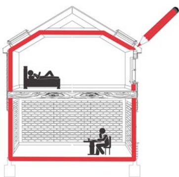
Figura 5.3: Discontinuidad hermética por cambio de material.
