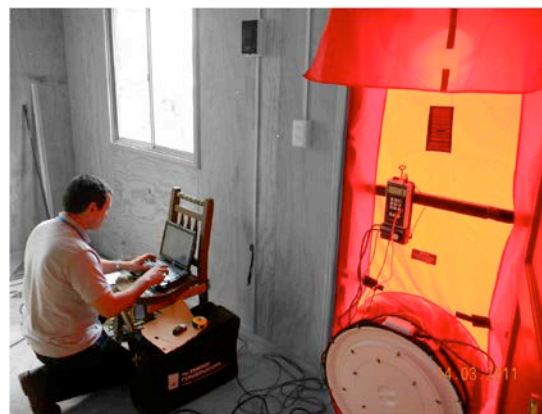
Figura 4.5: Ensayo de Blower Door.
