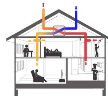
Figura 9.12: Esquema de ventilación con recuperador de calor
