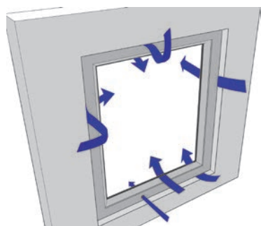
Figura 8.11: Principales puntos de infiltración de aire en ventanas fijas.
