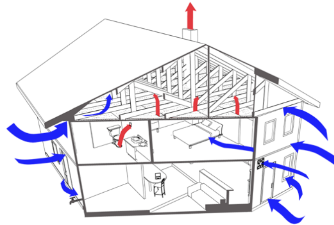
Figura 5.1: Puntos singulares de infiltración típicos de una construcción.
