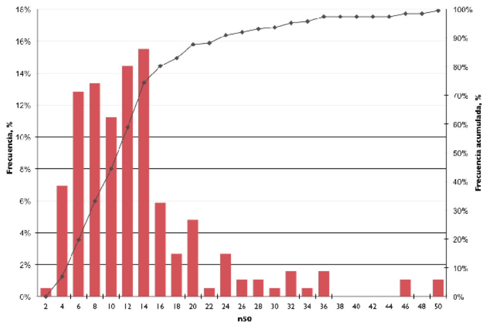
Figura 2.6: Frecuencia y frecuencia acumulada de valores de hermeticidad (n50) de la muestra ensayada.
