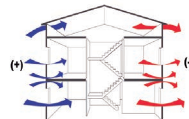
Figura 1.5: Esquema de infiltración producida por el viento.
