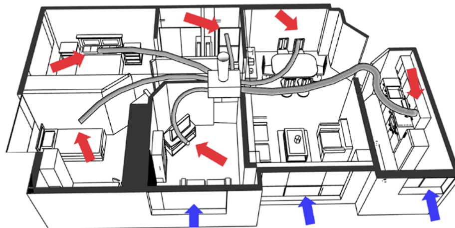
Figura 9.14: Esquema de ventilación natural convectiva
