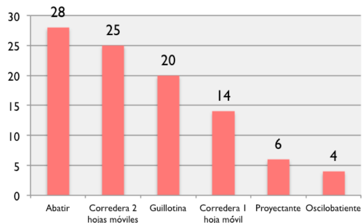
Figura 6.8: Infiltraciones de aire a 100 Pa por tipo de apertura de ventanas (m³/h m²).
