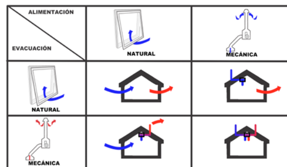
Figura 9.17: Tipos de alimentación y evacuación de aire
