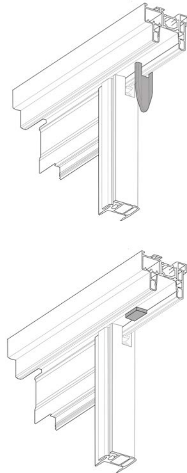
Figura 4.15: Tipos de topes estanco en ventanas correderas.
