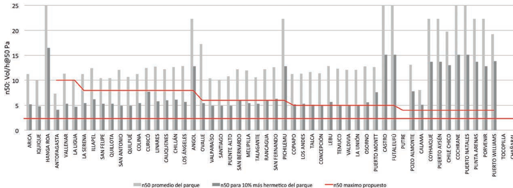
Figura 3.3: Brecha entre los valores límite y el 10% más hermético por localidad.
