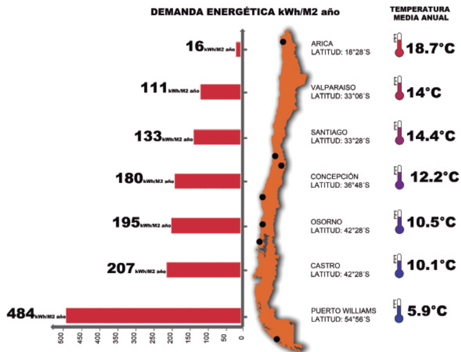
Figura 1.4: Demanda de energía actual calculada, De (kWh/m 2 año), para el acondicionamiento térmico de una vivienda típica de albañilería en las distintas zonas térmicas de Chile.
