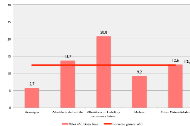
Figura 2.5: Línea base de la hermeticidad al aire promedio según materialidad predominante en muros para la edificación terciaria.
