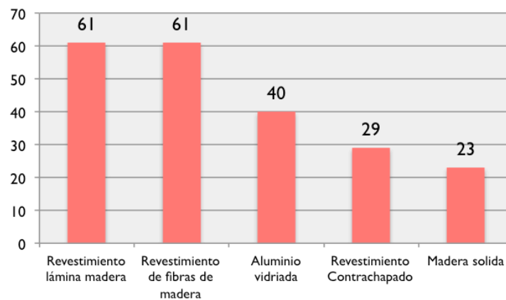
Figura 6.9: Infiltraciones de aire a 100 Pa por materialidad de puerta.
