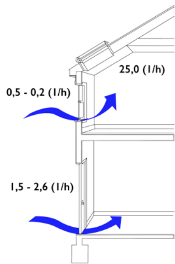
Figura 6.2: Infiltración de aire en ventanas y puertas en viviendas de hormigón armado.
