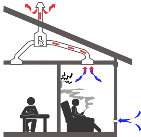
Figura 9.16: Esquema de ventilación híbrida
