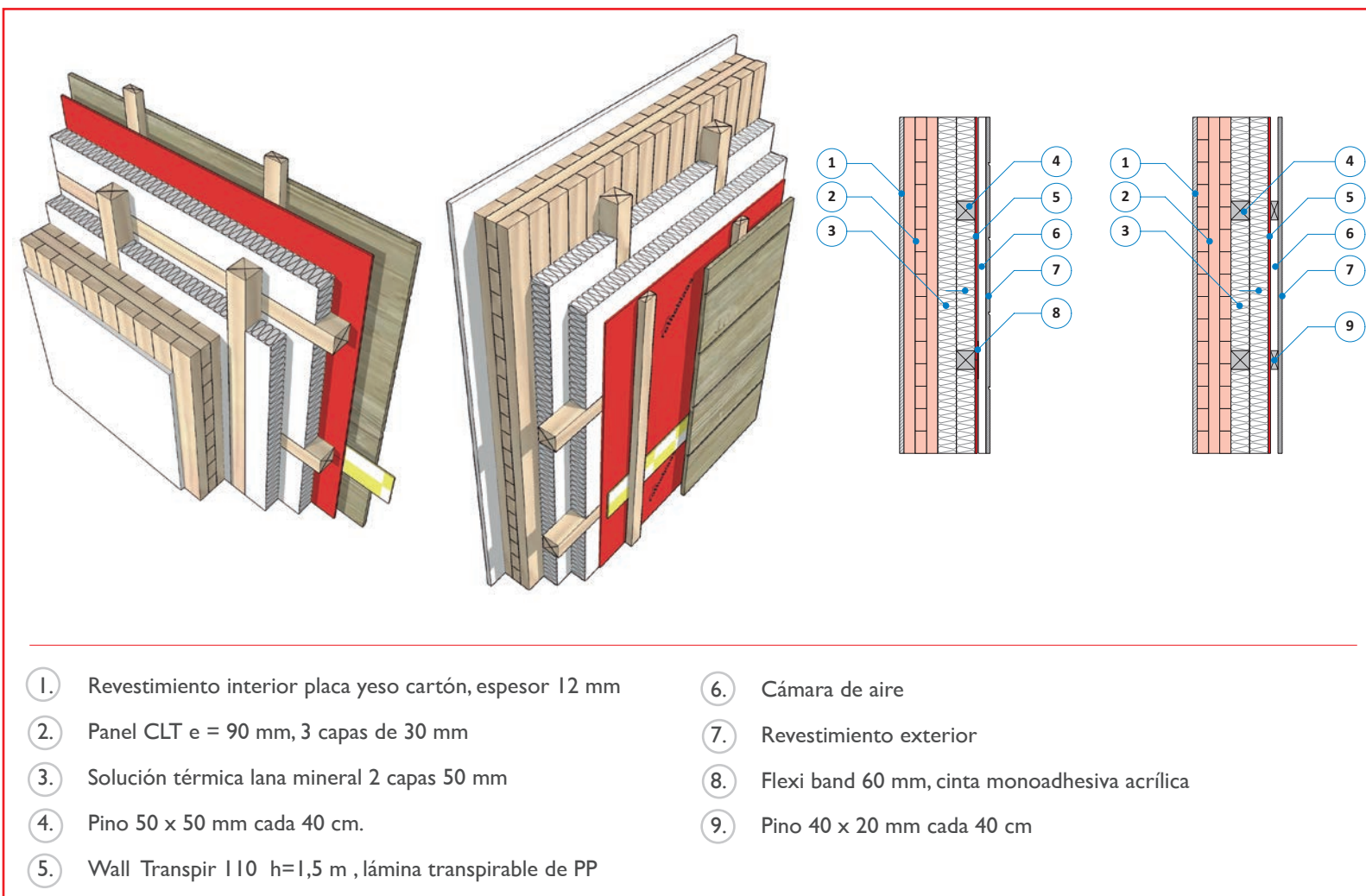
Figura 10.23: Detalle de muro envolvente
