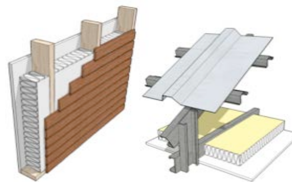
Figura 5.4: Sistema constructivo liviano.
