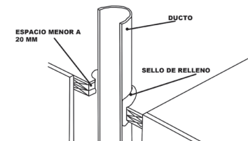
Figura 8.18: sello de relleno en ductos.
