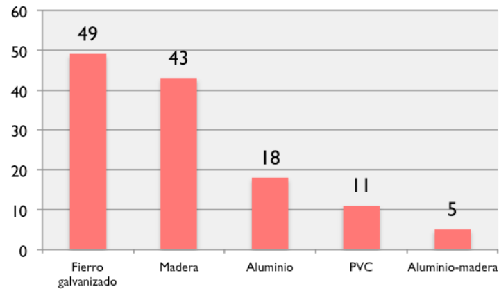
Figura 6.7: Infiltraciones de aire promedio a 100 Pa por materialidad de ventanas (m³/h m²).
