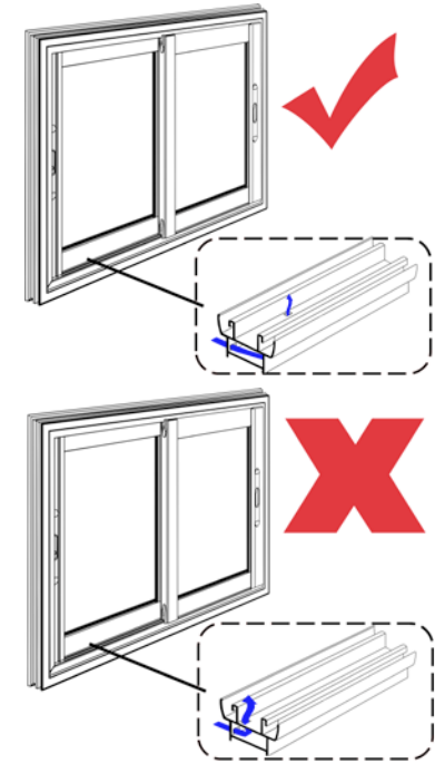
Figura 4.13: Desfase de perforaciones de desagües entre el exterior e interior de una ventana.
