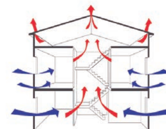
Figura 1.6: Esquema de infiltración por efecto de diferencia de temperatura.
