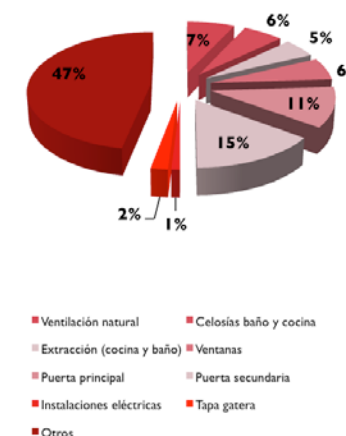
Figura 5.9: Incidencia de puntos singulares a la hermeticidad al aire en sistema pesado.
