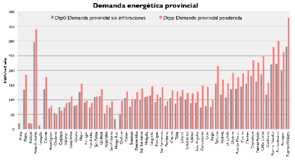
Figura 1.9: Demanda energética de viviendas en cada capital provincial ponderada por tipologías constructivas. Demanda sin considerar infiltraciones y considerando infiltraciones.
