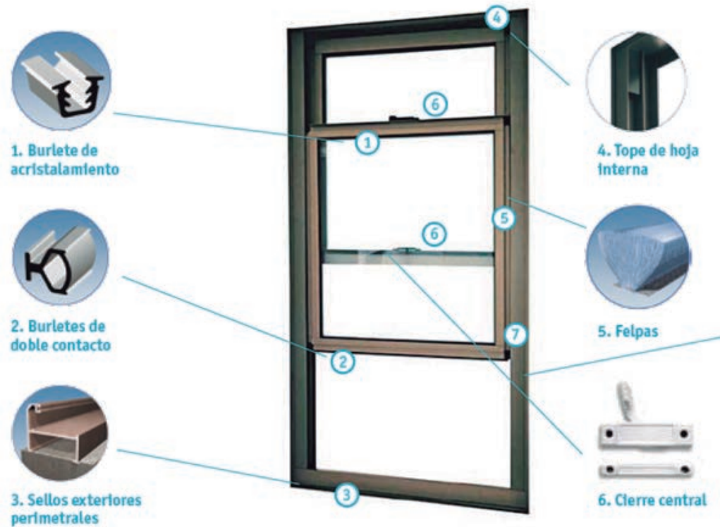
Figura 7.10: Ejemplo de ubicación de los diferentes sellos que son necesarios en la fabricación de una ventana de guillotina. (Fuente: documento técnico N° 28CDT-CCHC y CORFO).
