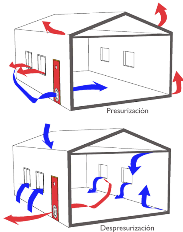
Figura 4.8: Presurización y despresurización de recinto.
