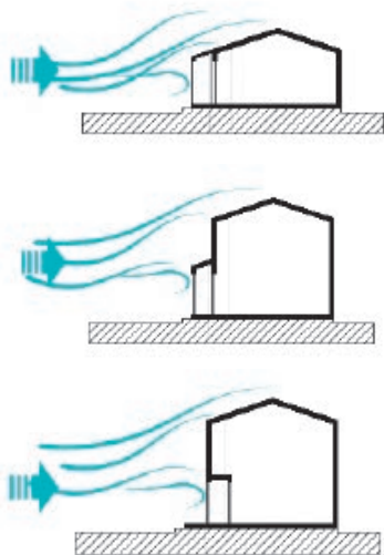
Figura 8.2: Diagramas de chifloneras.
