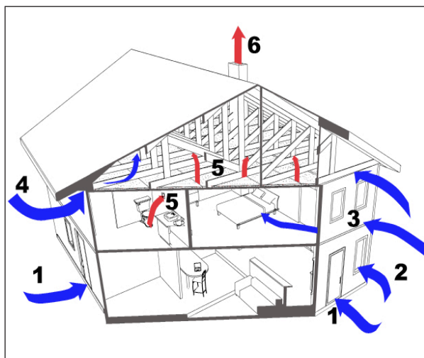
Figura 1.8: Principales vías de ocurrencia de infiltraciones de aire.
