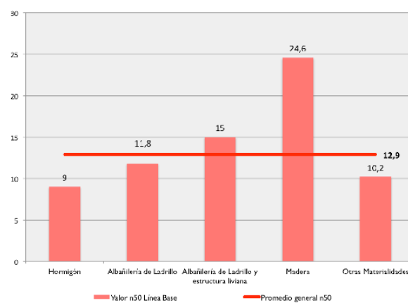
Figura 2.4: Línea base de hermeticidad al aire promedio según materialidad predominante en la envolvente para la edificación habitacional.
