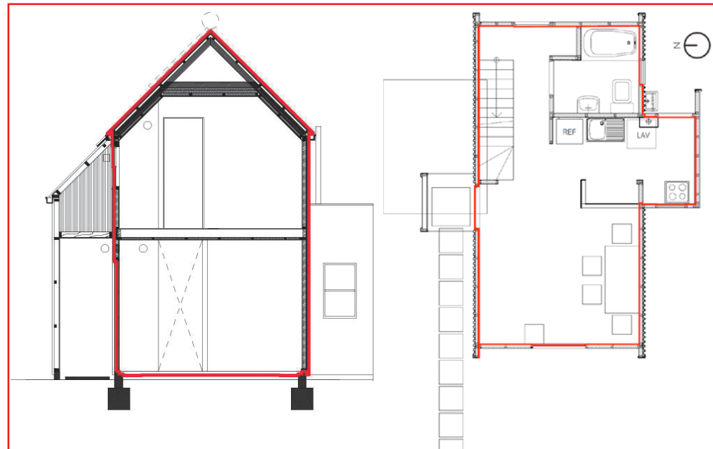
Figura 10.7: Esquema de la línea roja en la envolvente de la vivienda
