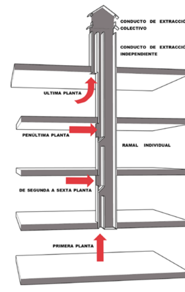
Figura 9.7: Sistema de extracción colectiva. En caso de utilizar este sistema no debe servir a más de 6 plantas. Si existieran, los ductos de plantas sobre ese nivel deberían ser individuales.
