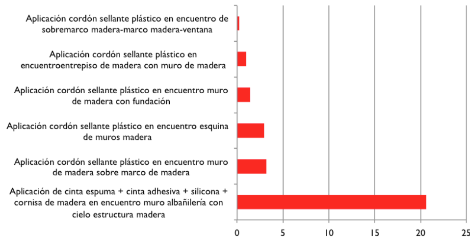
Figura 5.8: Reducción de la permeabilidad al aire mediante la aplicación de técnicas de sellado por metro lineal de junta.
