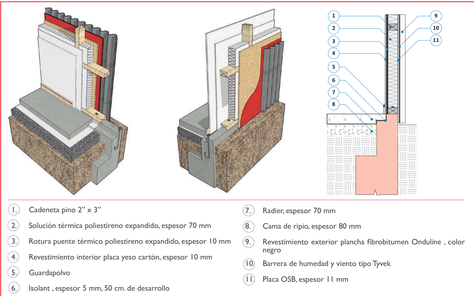
Figura 10.9: Detalle encuentro muro y fundación
