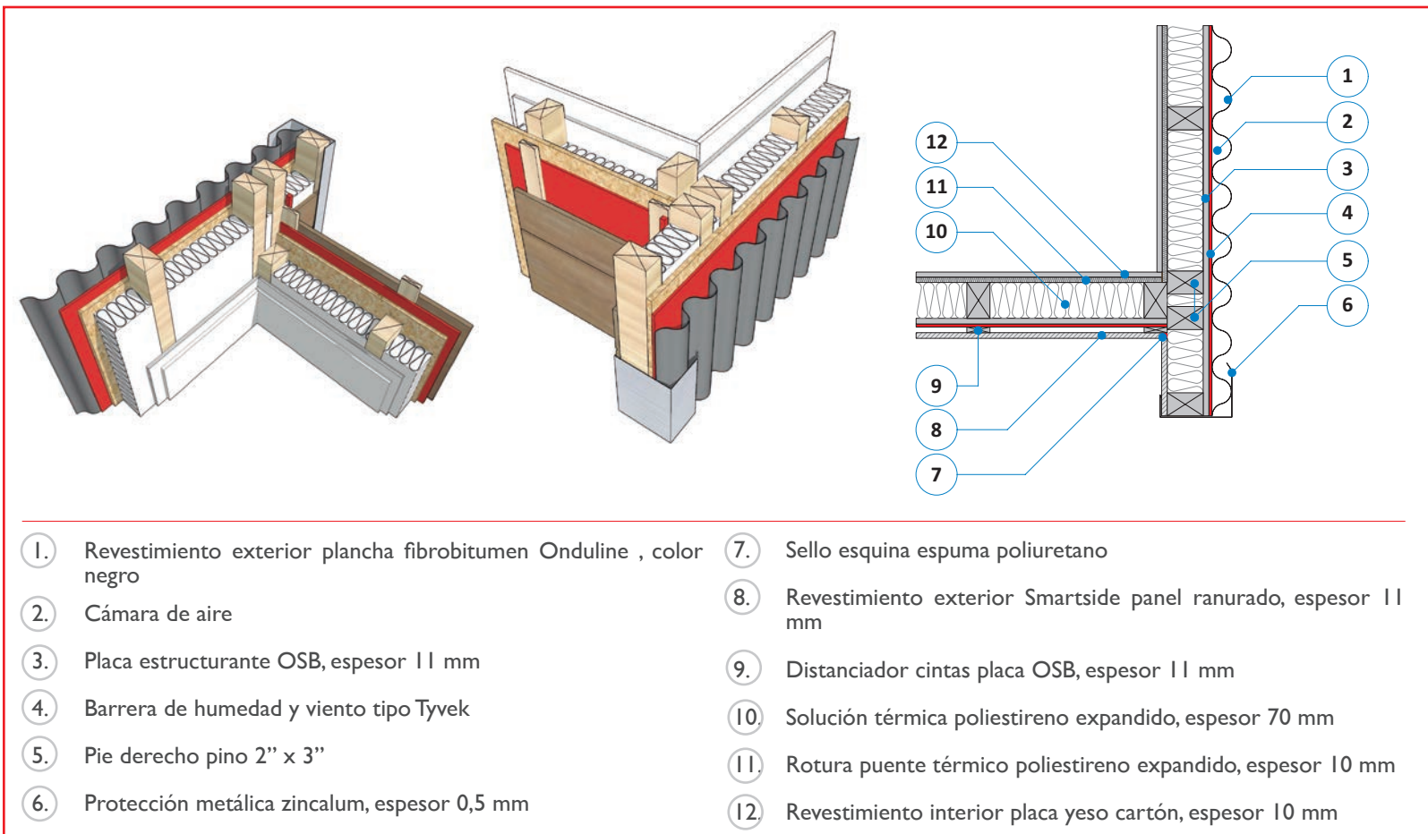
Figura 10.8: Detalle de encuentro de muros
