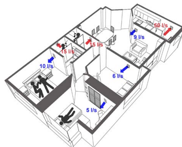
Figura 9.6: Ejemplo de caudales de ventilación para cada recinto de una vivienda
