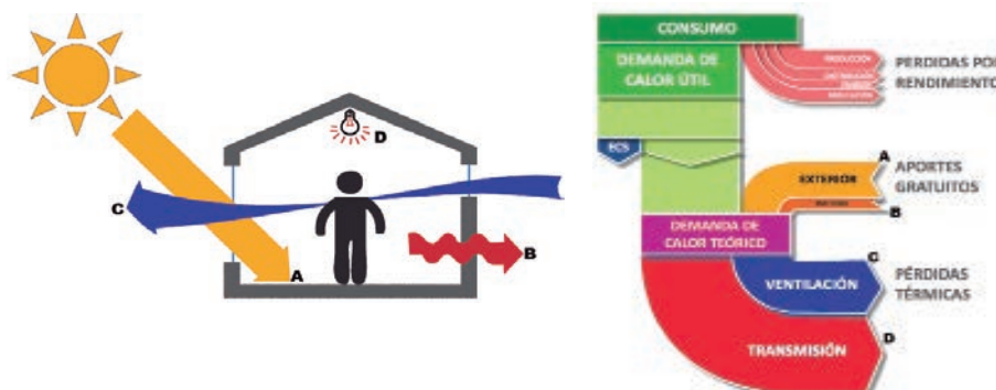
Figura 1.2: Ganancias y pérdidas de calor y diagrama del balance energético de un edificio tipo en régimen de calefacción.
