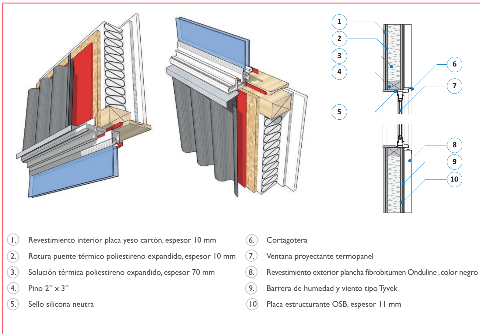
Figura 10.12: Detalle encuentro muro - ventana
