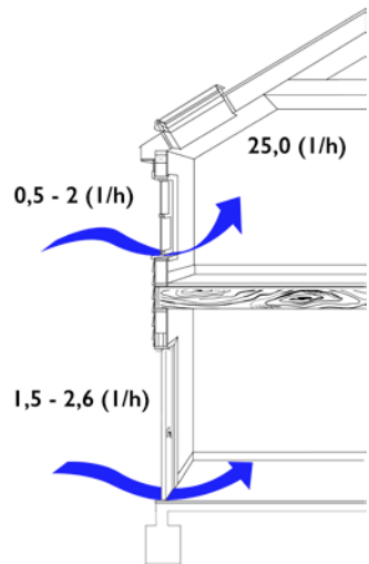
Figura 6.3: Infiltración de aire en ventanas y puertas en viviendas de madera.
