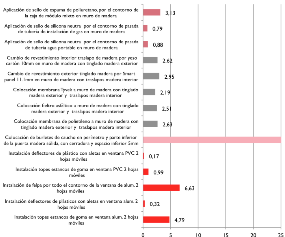
Figura 5.7: Reducción de la permeabilidad al aire mediante la aplicación de técnicas de sellado por unidad de superficie.
