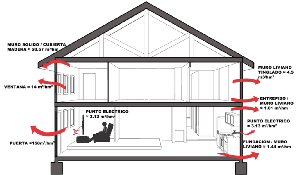
Figura 5.12: Reducción de la permeabilidad al aire mediante la aplicación de técnicas de sellado por metro lineal de junta.
