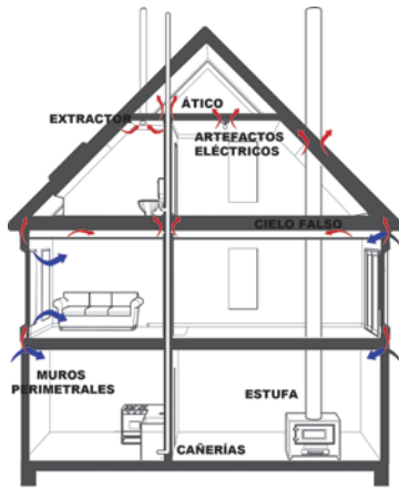
Figura 8.16: Puntos de fuga de aire en ductos de instalaciones
