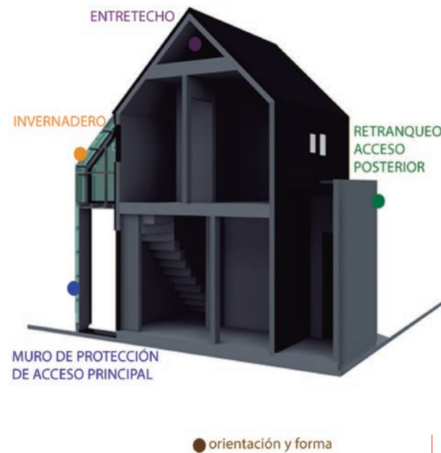
Figura 10.15: Esquema en corte
